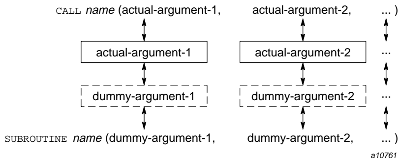
Figure 10. Actual and dummy argument lists
