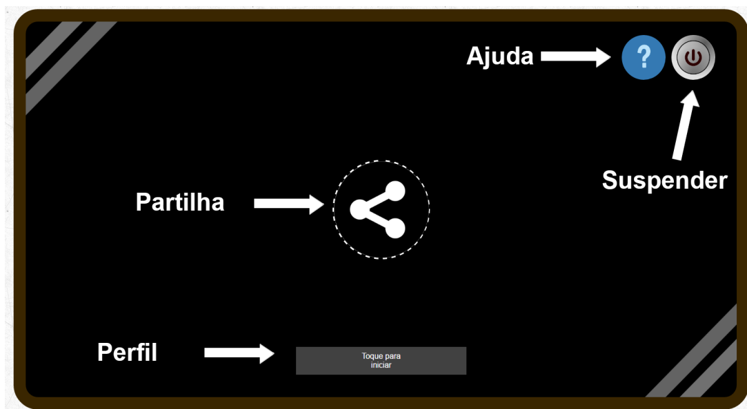
Figura 2: Ecrã principal
