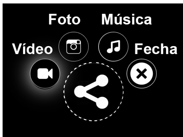
Figura 13: Botão Vídeo
