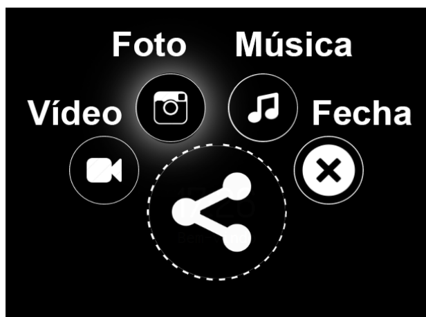
Figura 16: Botão Foto
