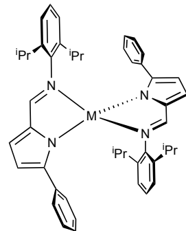
[M(L2) 2 ]
